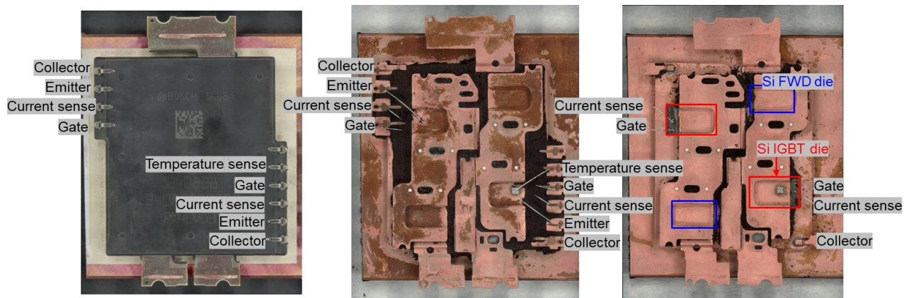
モジュール内部レイアウト
