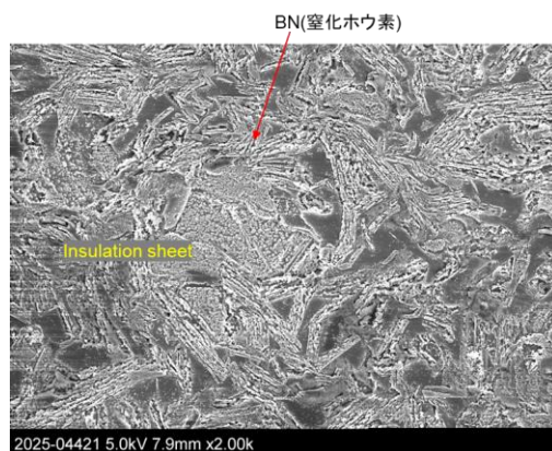
絶縁シート 拡大断面SEM像
