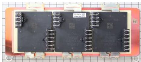
Si IGBTモジュール外観
