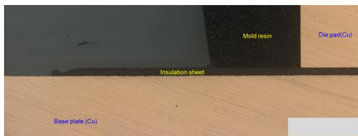
絶縁シート断面OM像
