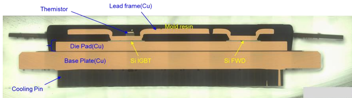
モジュール断面
