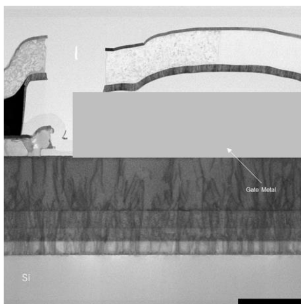
セル領域 断面TEM像 (GaN-Epi層)
