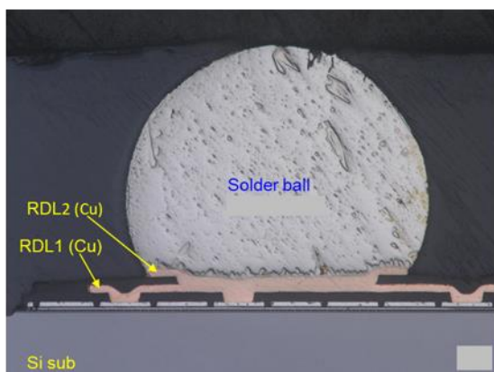
パッケージ断面構造
