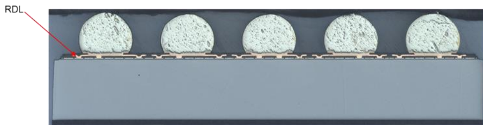
パッケージ断面構造
