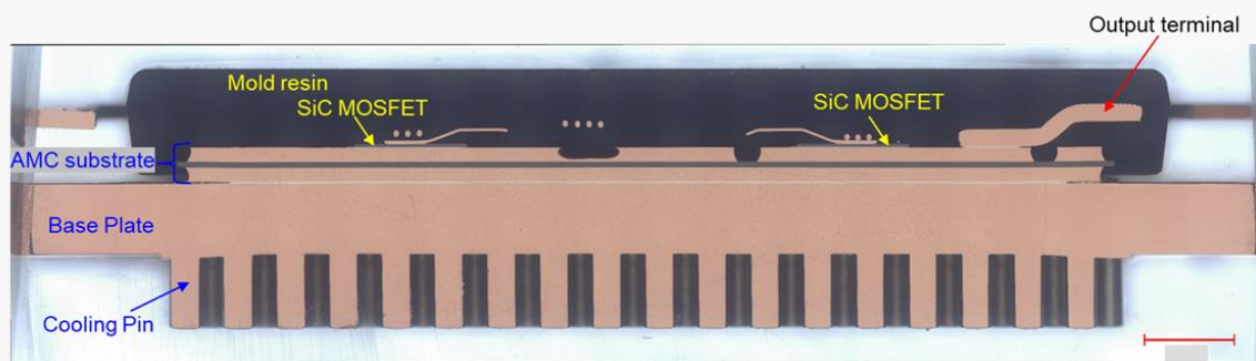
モジュール断面 全体像
