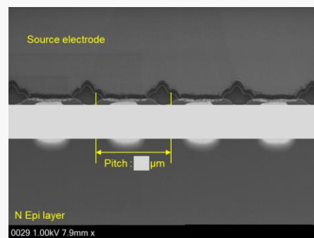
セル部 断面SEM像
