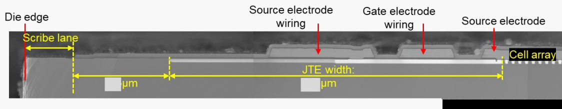
チップ外周部 断面SEM像
