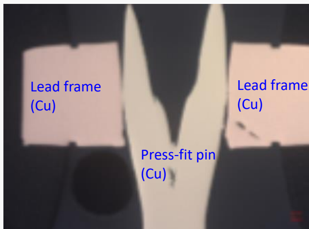
プレスフィット端子 断面像
