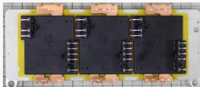
UAES製 パワーモジュール×3相
