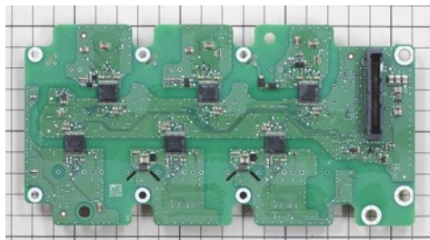
搭載ゲートドライブ基板
