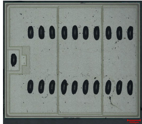
チップ外観
