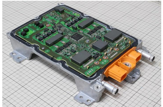
搭載DCDCコンバータ基板
