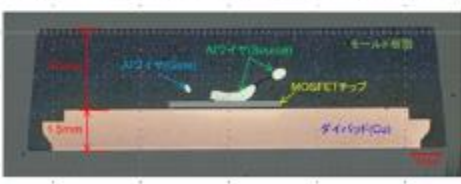
パッケージ断面
