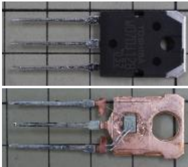
パッケージ写真
