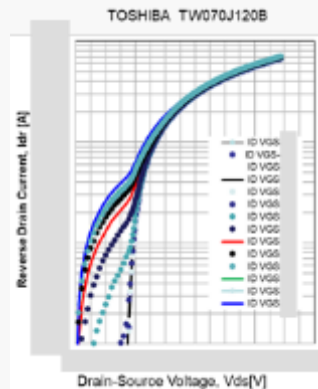
Fig. 4-5-1 逆ドレイン電流(ショットキーダイオード)特性のゲート電圧(VGS)依存性
