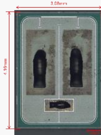
チップ写真
