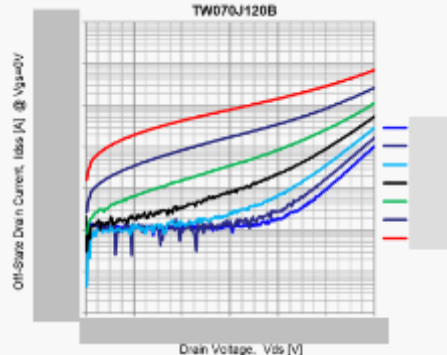
Fig. 4-2-1 デバイス温度をパラメータとしたオフ状態のIdss-Vds特性
