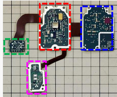
センサ基板 (Top View)
