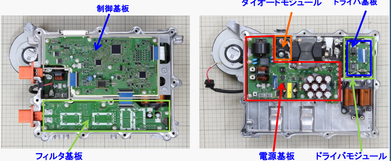
製品内観制御基板
