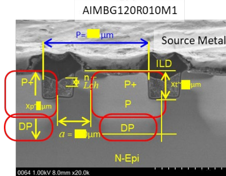
Fig. 1-6-1 トランジスタセル
