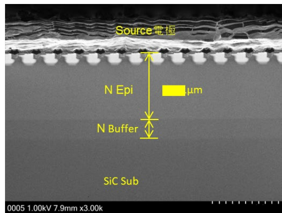
N Epi層膜厚 断面SEM像
