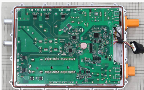
NetPower製OBC(CA16K6-2AL)内部
